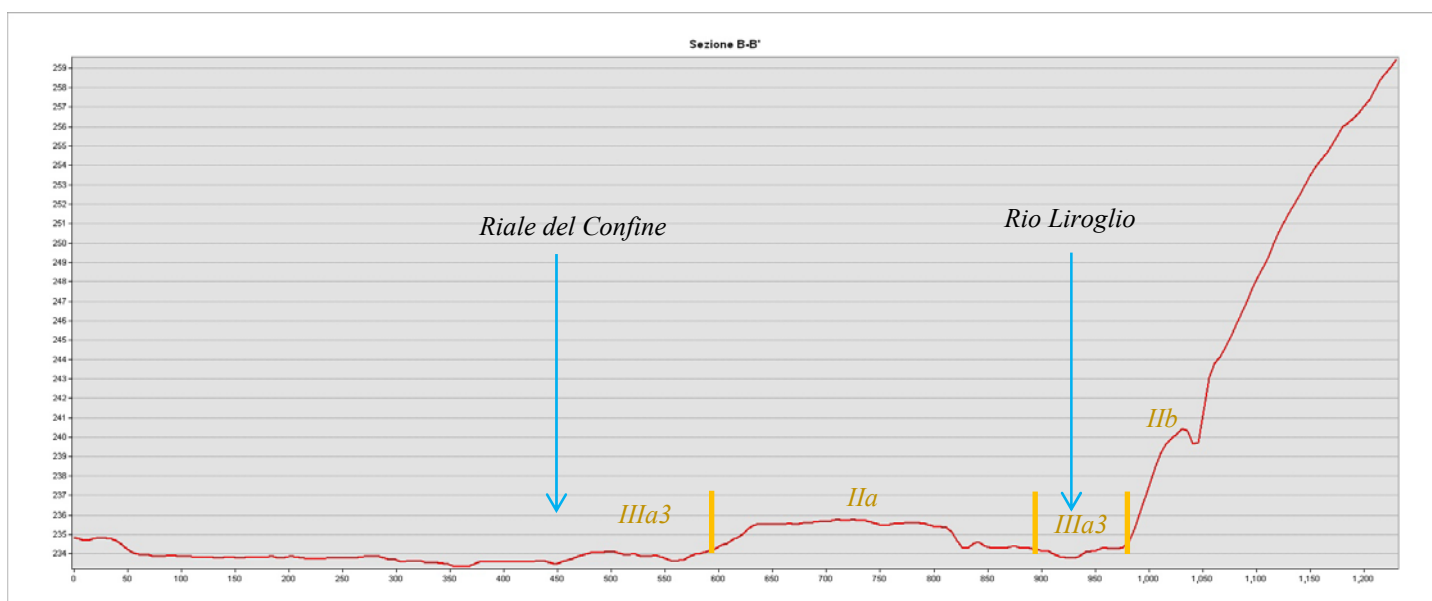
Fig.3: sezione topografica B-B' con rappresentazione dei principali corsi d'acqua e limiti tra le classi di sintesi
