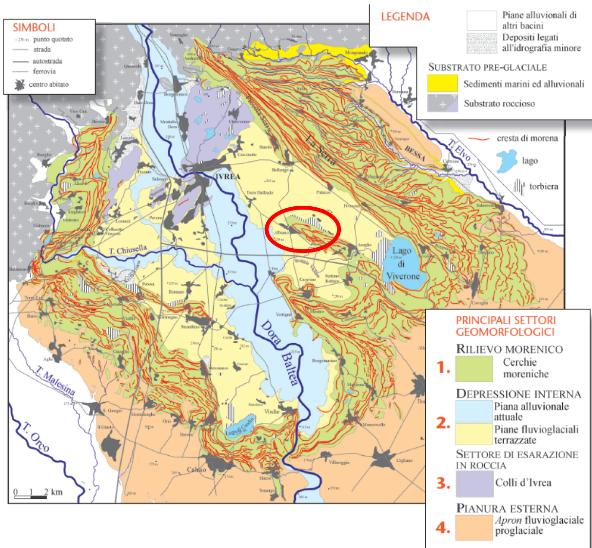
Fig. 2: Carta dei principali settori geomorfologici dell'Anfiteatro Morenico di Ivrea (Gianotti, 2007)
