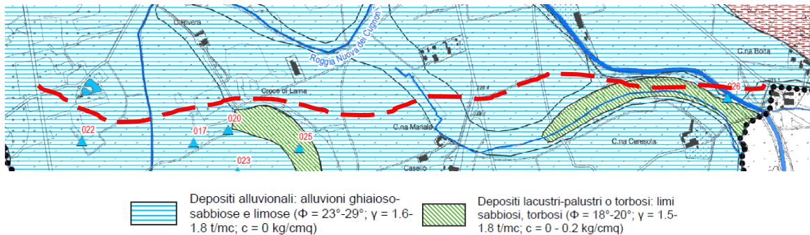
Estratto Tav. 06 "Carta litotecnica", allegata al P.R.G.C. (aprile 2025)
