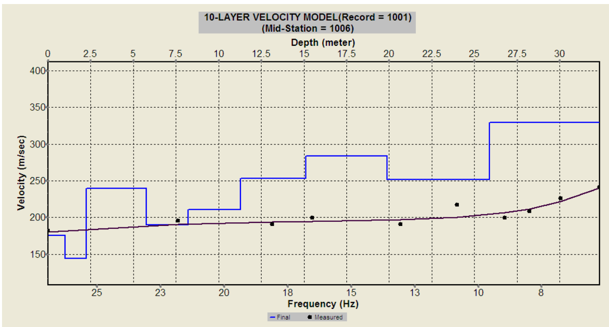
Profilo stratigrafico monodimensionale delle Vs
