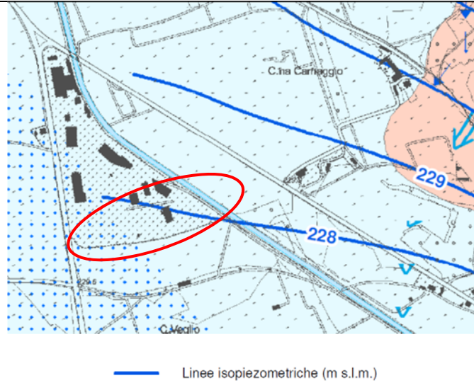
Estratto Tav. 03 “Carta geoidrologica”, allegata al P.R.G.C. (aprile 2025)
