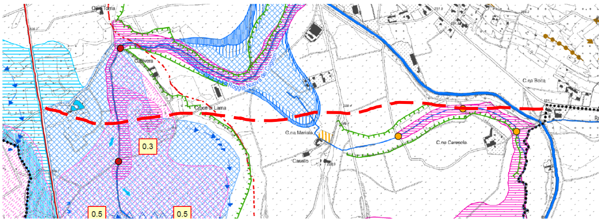
Estratto Tav. 02A “Carta geomorfologica e idraulica”, allegata al P.R.G.C. (aprile 2025)
