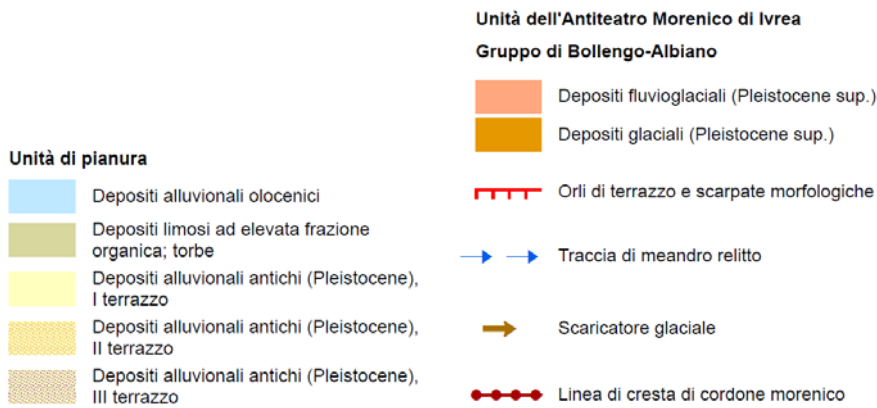
Estratto Tav. 01 "Carta geologic-strutturale", allegata al P.R.G.C. (aprile 2025)
